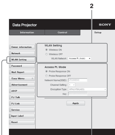
Кнопка WLAN Setting 3-(a)
