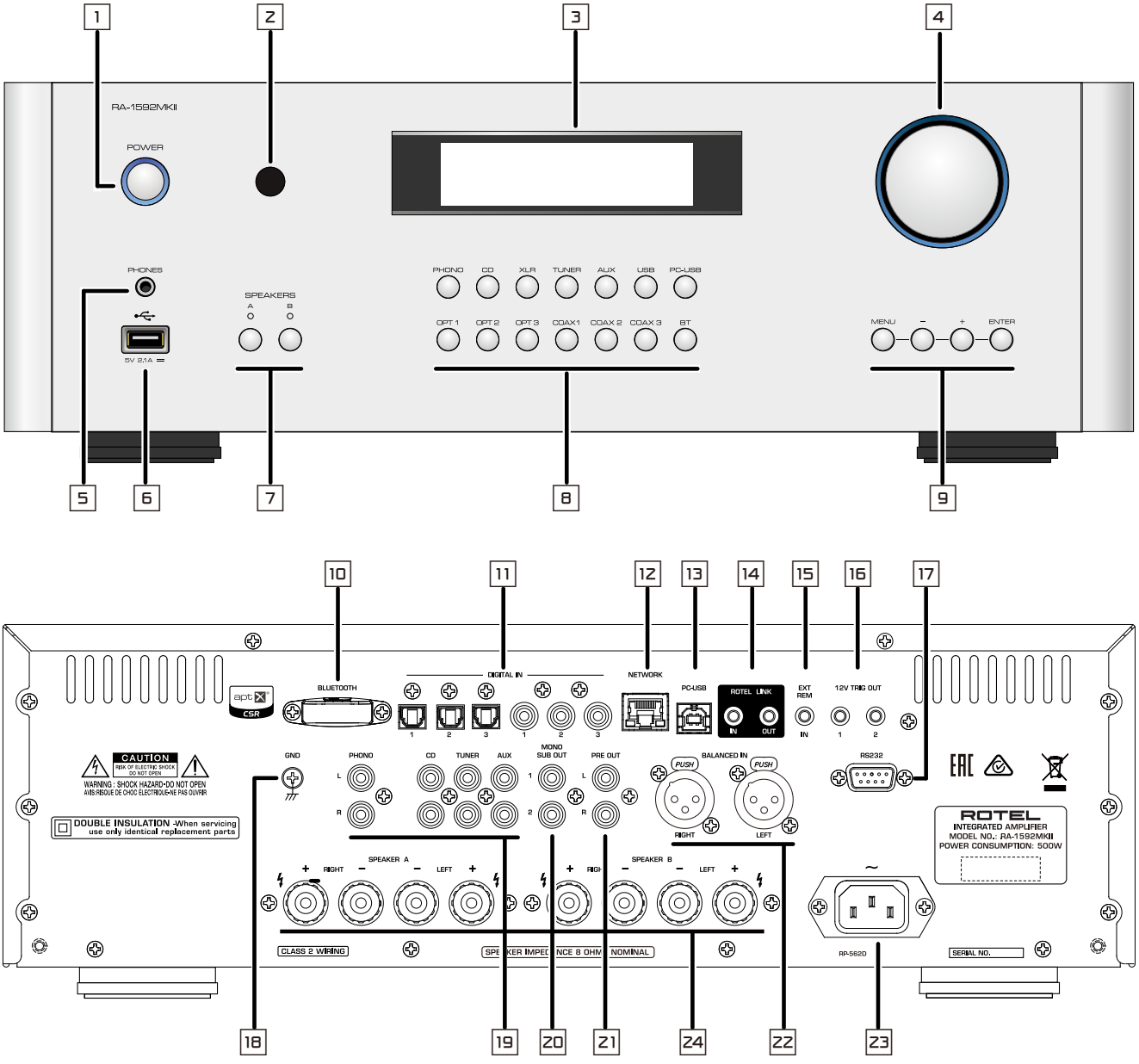
Figure 1: Controls and Connections Commandes et Branchements Bedienelemente und Anschlüsse Controlles y Conexiones Bedieningselementen en aansluitingen Controlli e connessioni Controller och anslutningar Органы управления и разъемы
