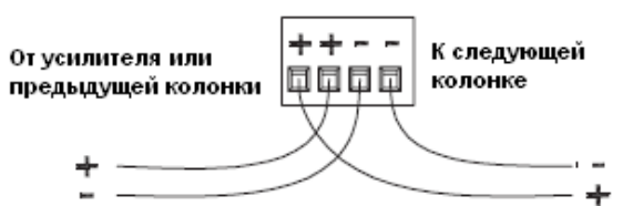
Рисунок 13. Последовательное подключение
