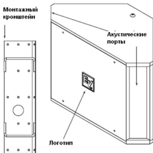
Рисунок 18. Вид спереди.
