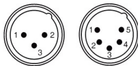
Ввод данных DMX Вилки XLR (вид сзади)
