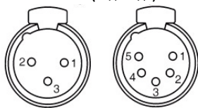
Использование разъема XLR для вывода данных DMX Разъемы XLR (вид сзади)
