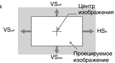
Затемненная область: диапазон сдвига объектива
