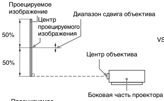
Затемненная область: диапазон сдвига объектива
