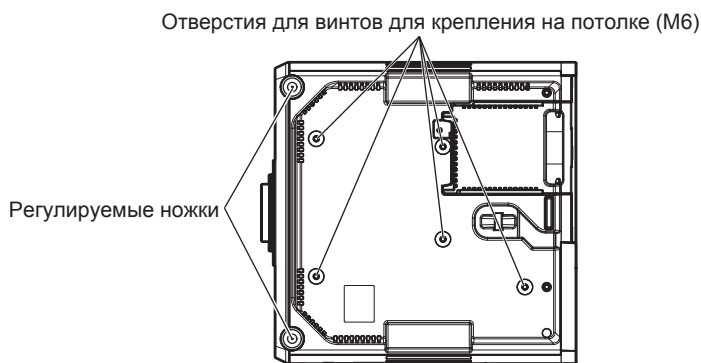
Положения отверстий для винтов для крепления на потолке и регулируемых ножек
