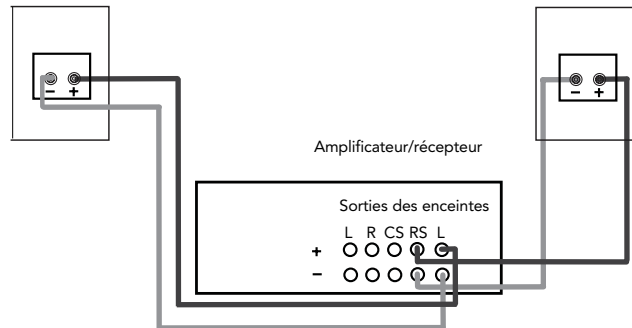
FIGURE 3 – RACCORDEMENT DE L'ENCEINTE À L'AMPLIFICATEUR
