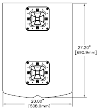
Вид сверху
