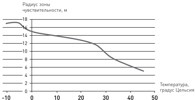
Рис.1. График зависимости радиуса зоны чувствительности от температуры.
