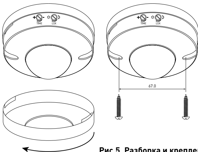
Рис.5. Разборка и крепление корпуса.
