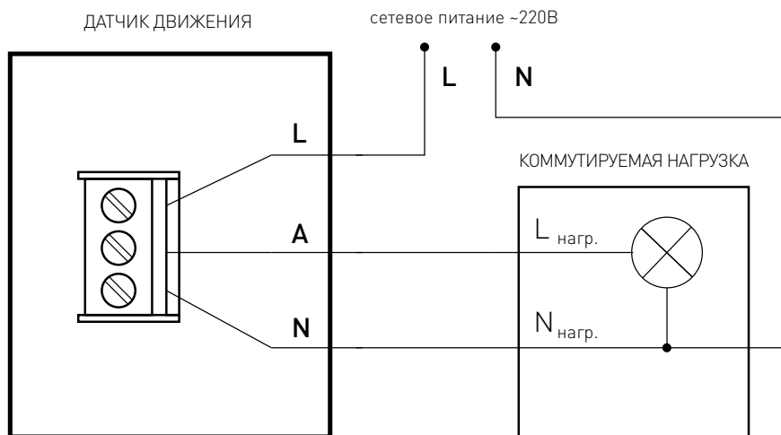
Рис.6. Подключение датчика движения.
