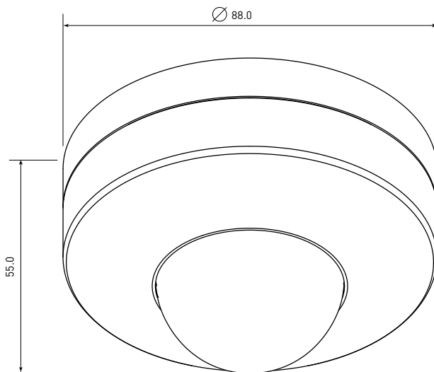
Рис.2. Габаритные размеры датчика движения.
