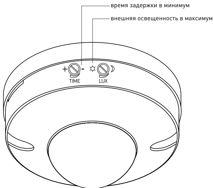
Рис.3. Начальные установки регуляторов во время настройки датчика.
