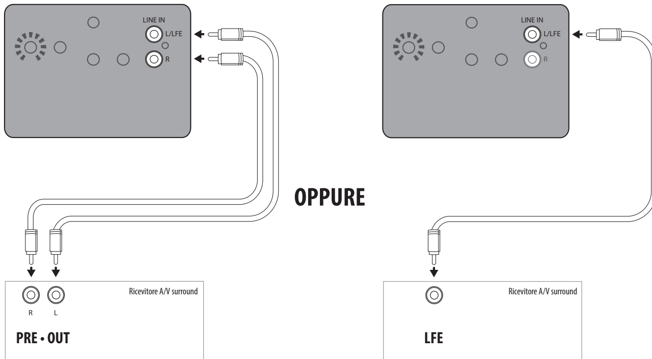
Figura 2 Connessioni Di Un Subwoofer J 110, J 112
