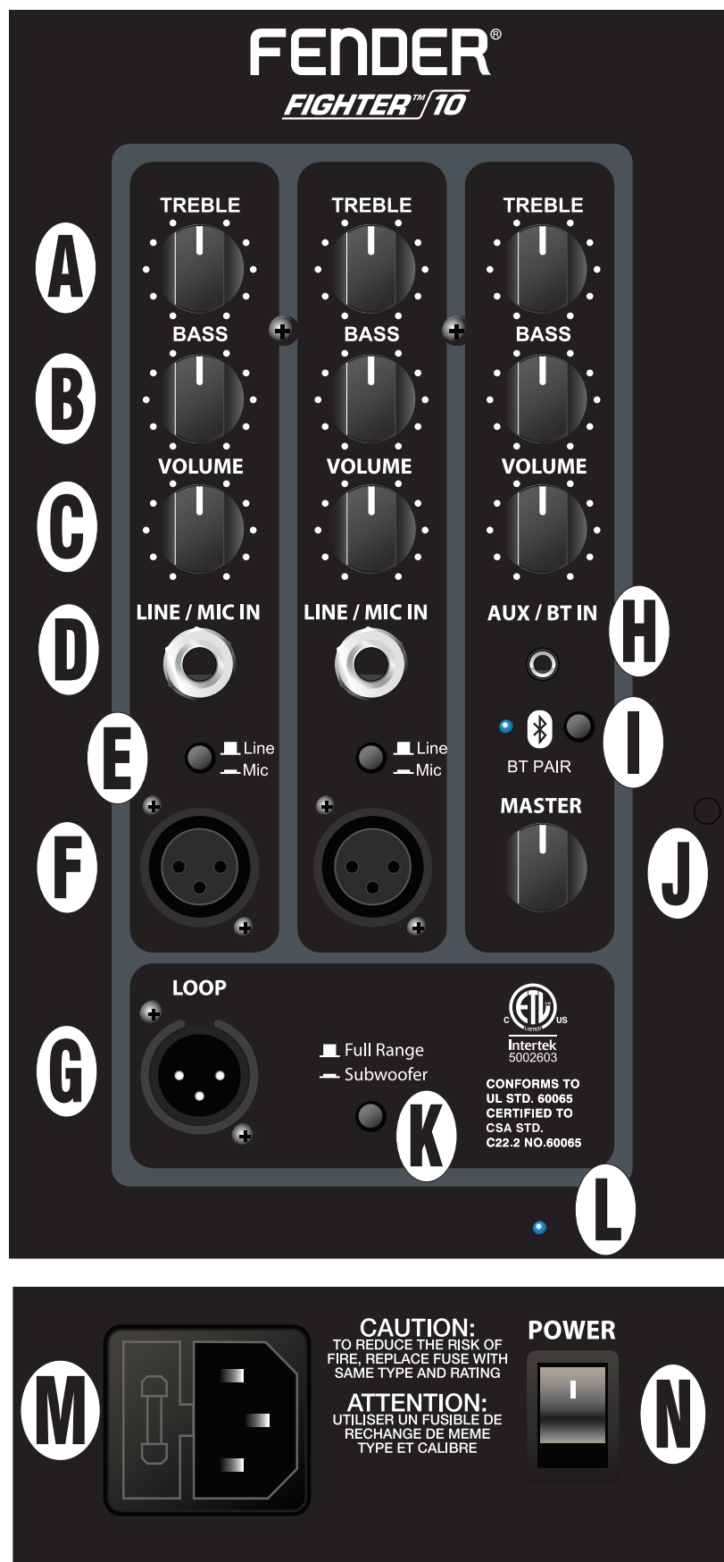
図は Fighter 10 背面パネル； Fighter 12 の機能およびレイアウトも同様です。
