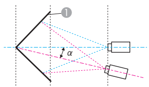
Вид сбоку
