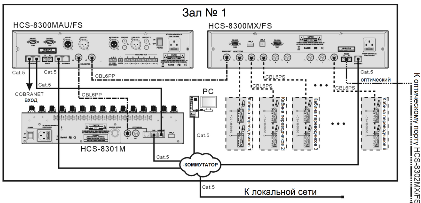
Рисунок 6.4.2 Соединение с конгресс-блоком синхронного перевода HCS-8300MX/FS
