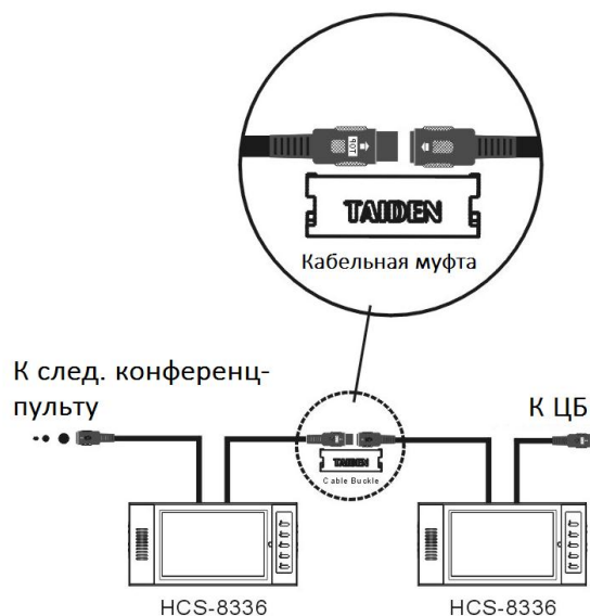
Рис. 3.4.5 Замкнутое гирляндное соединение между мониторами HCS-8336
