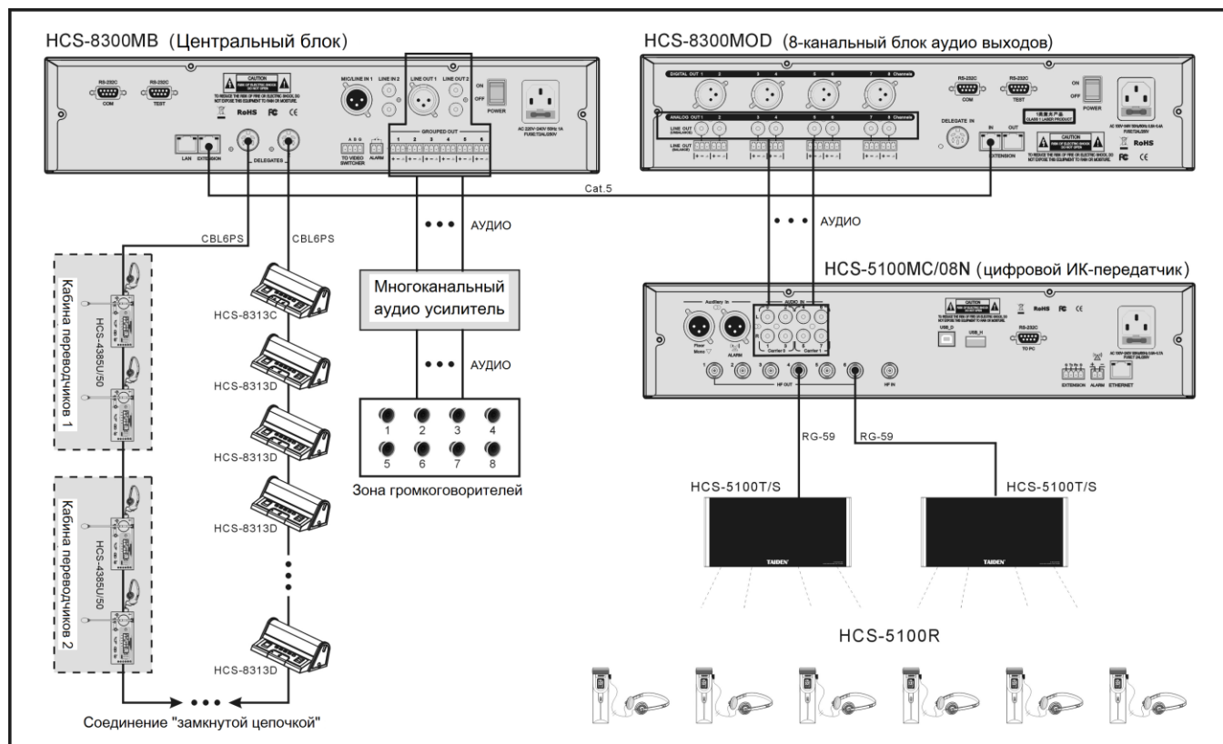
Рисунок 5.1.4 Центральный блок системы, соединенный с цифровой инфракрасной системой синхронного перевода через передатчик HCS-5100MC/N
