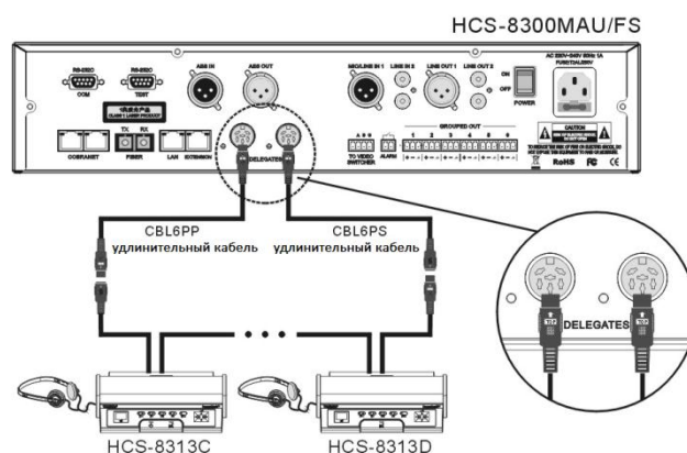
Рис. 3.2.3 Соединение «замкнутой петлей» между ЦБ и дискуссионными пультами серии HCS-8315
