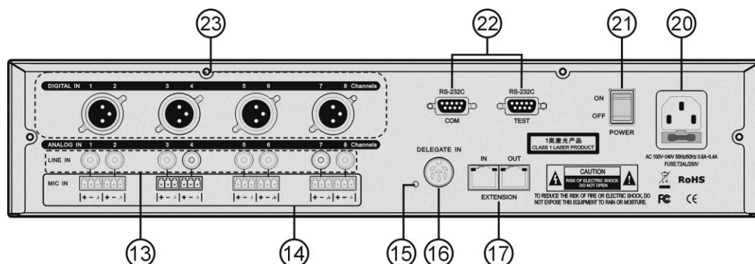
Задняя панель HCS-8300MID
