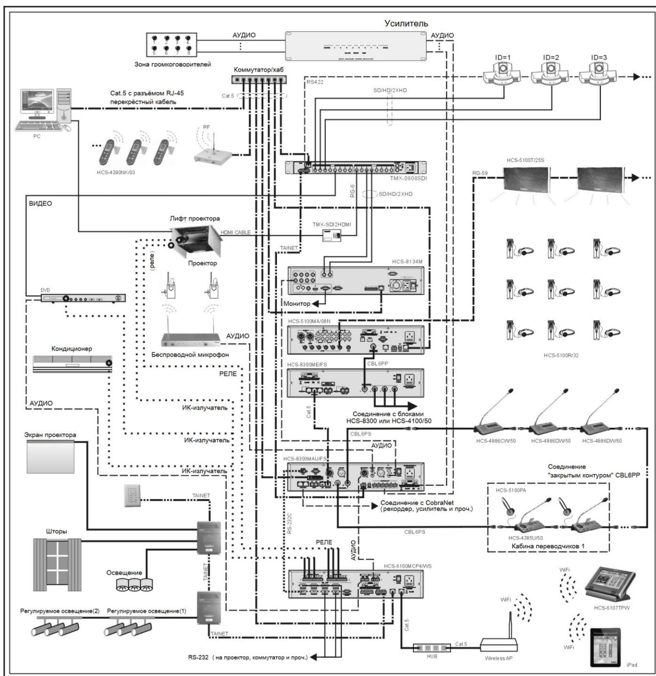
Рисунок 5.1.5 Соединение между конгресс-системой HCS-8300M и центральной системой управления
