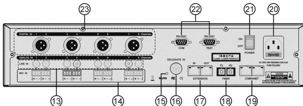
Задняя панель HCS-8300MID/FS
