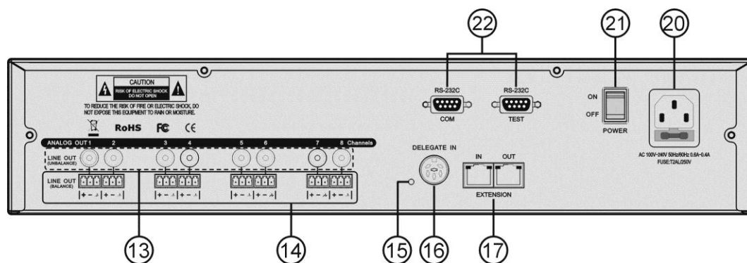
Задняя панель HCS-8300MOA
