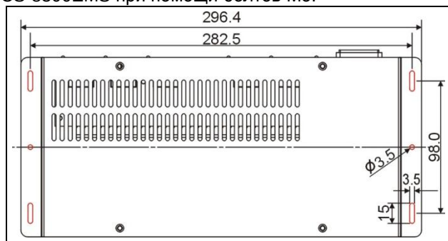
Рис 2.3.2 Монтаж блока HCS-8300EMS
