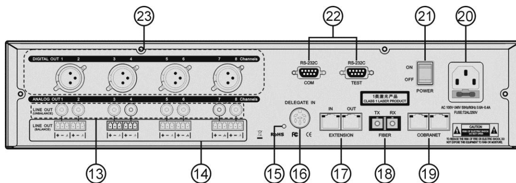
Задняя панель HCS-8300MOD/FS
