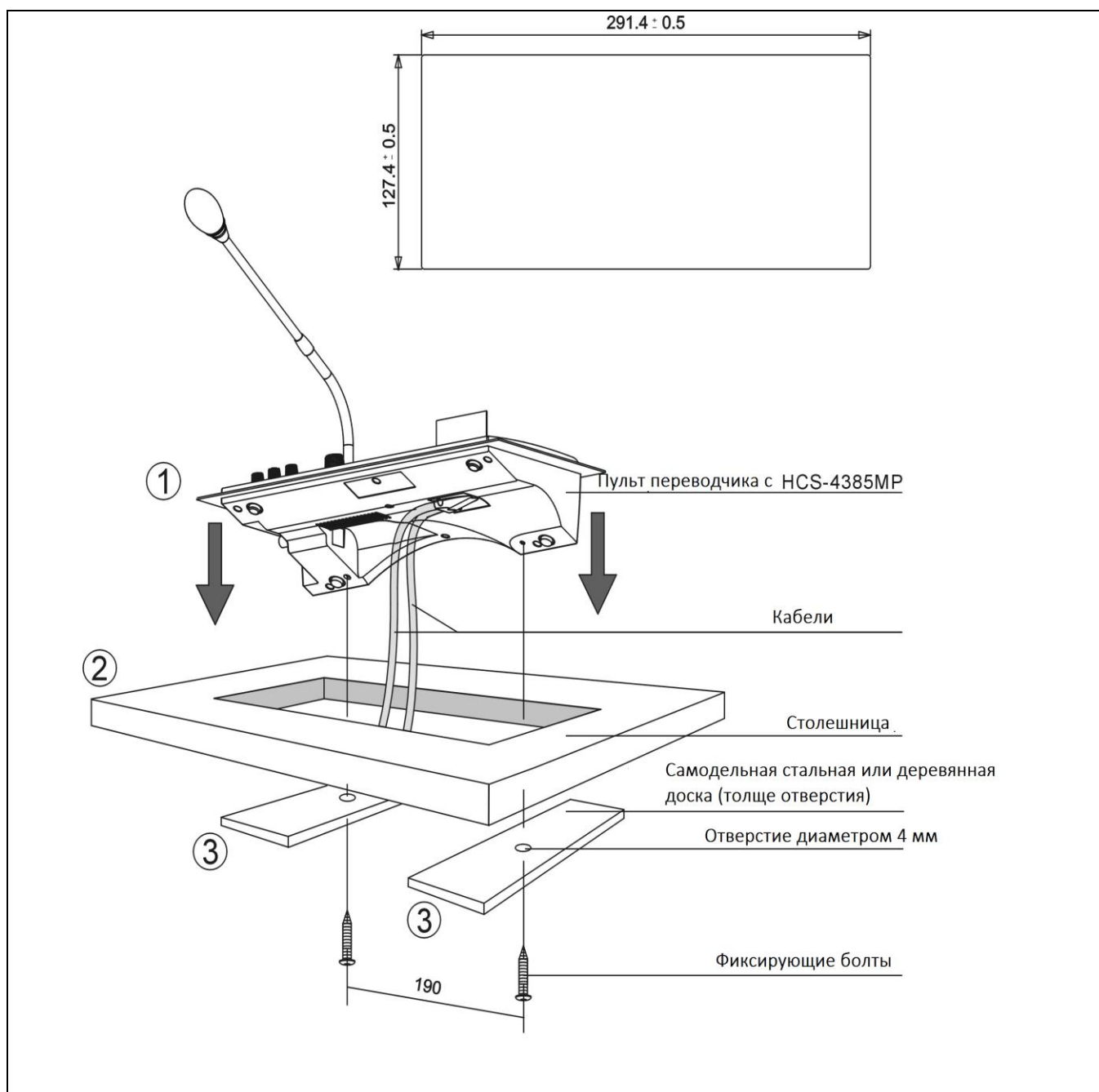
Рис. 4.2.1. Схема монтажа (пульт: мм)
