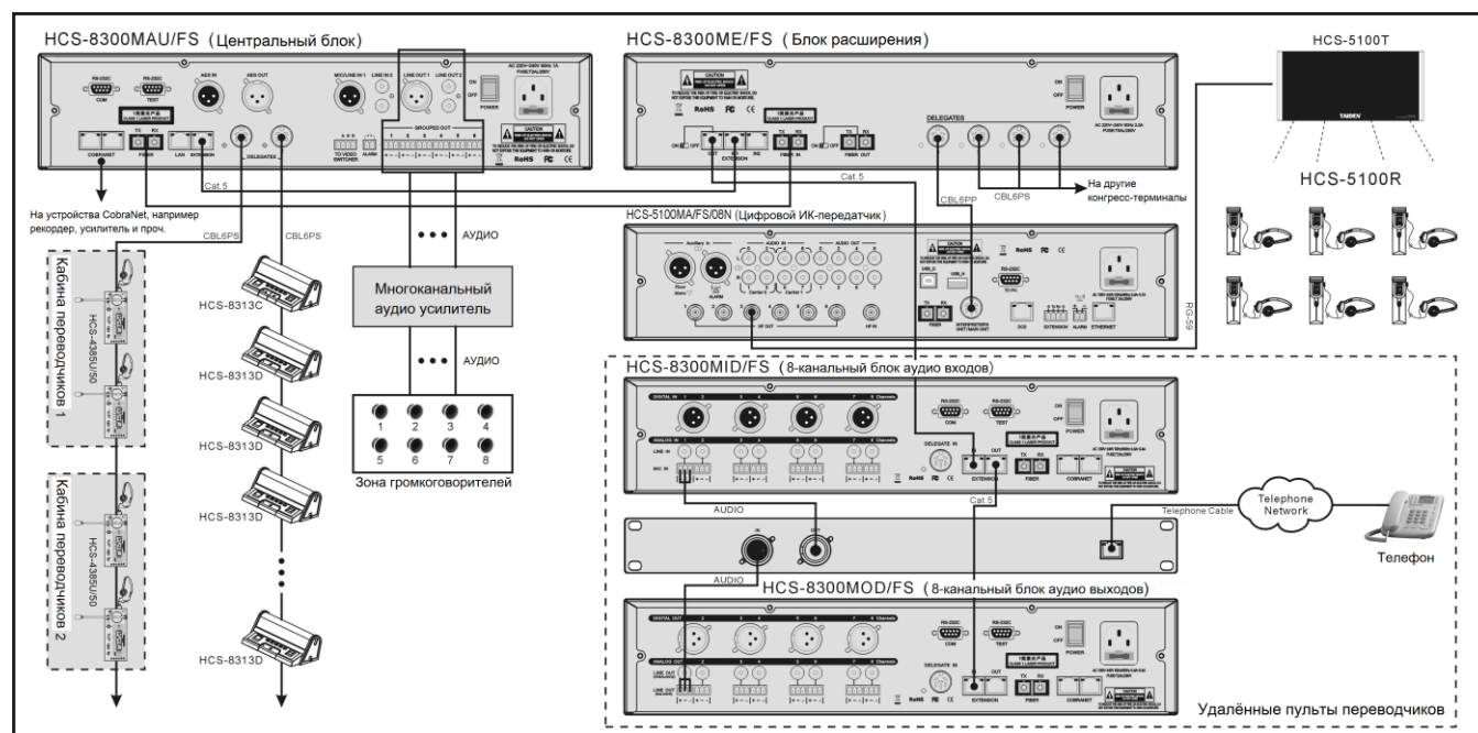
Рисунок 5.1.11 Система удалённого перевода
