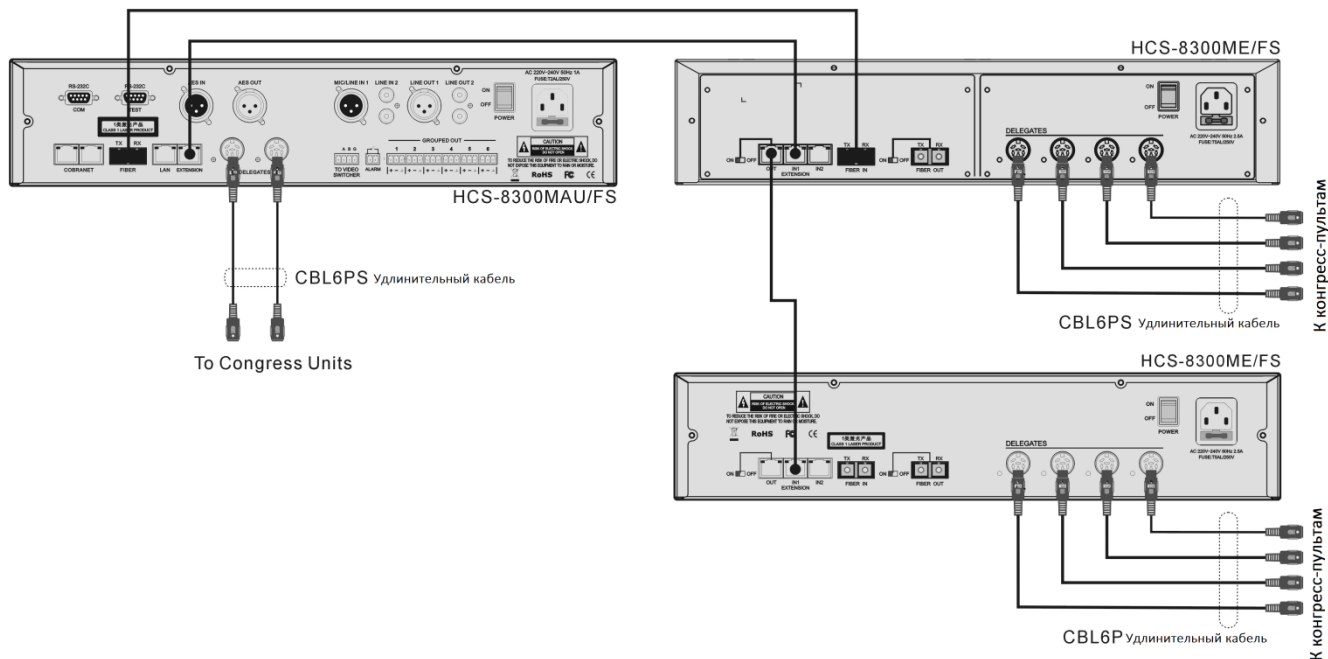
Рис. 2.2.4 Соединение между центральным блоком и блоками расширения
