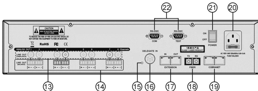
Задняя панель HCS-8300MOA/FS
