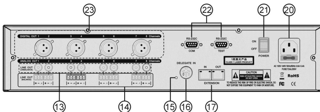
Задняя панель HCS-8300MOD
