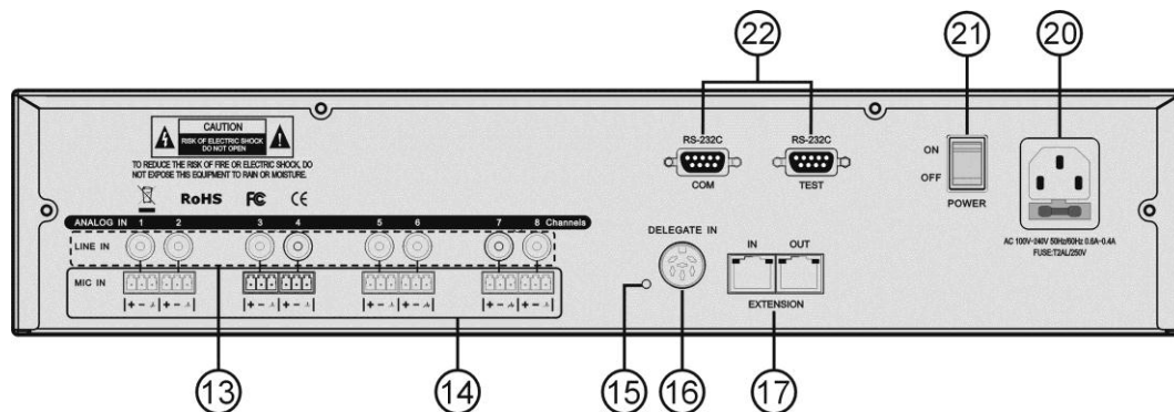
Задняя панель HCS-8300MIA
