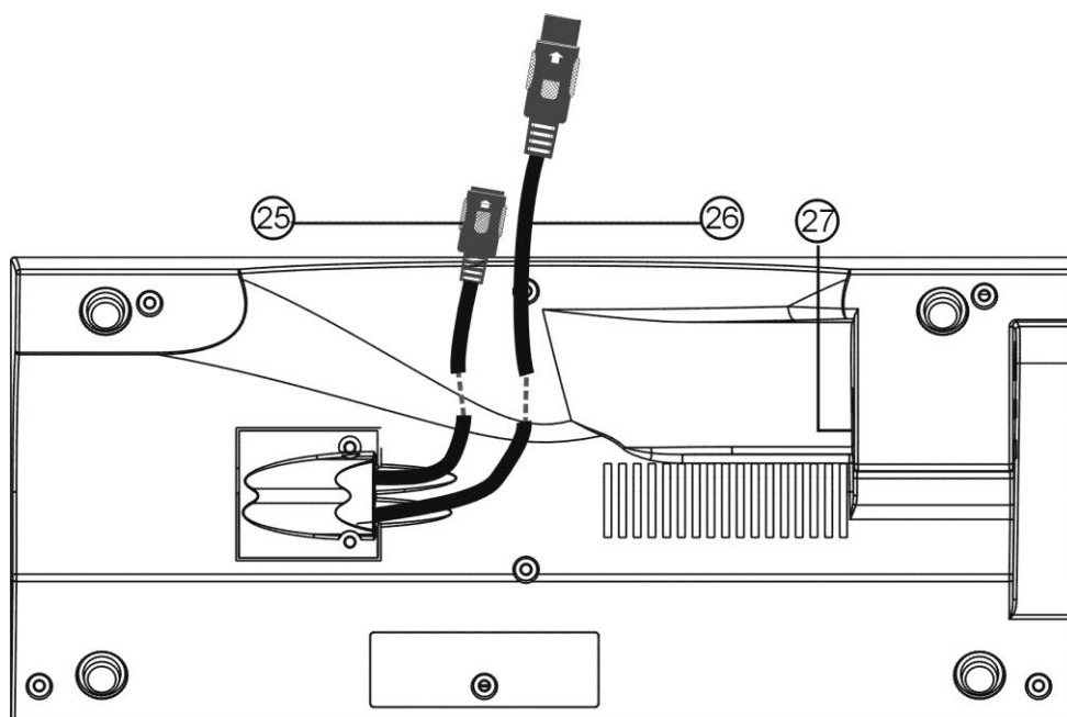
Задняя панель
