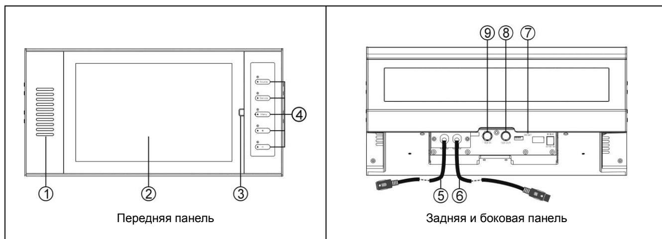
Рис. 3.4 Монитор HCS-8336
