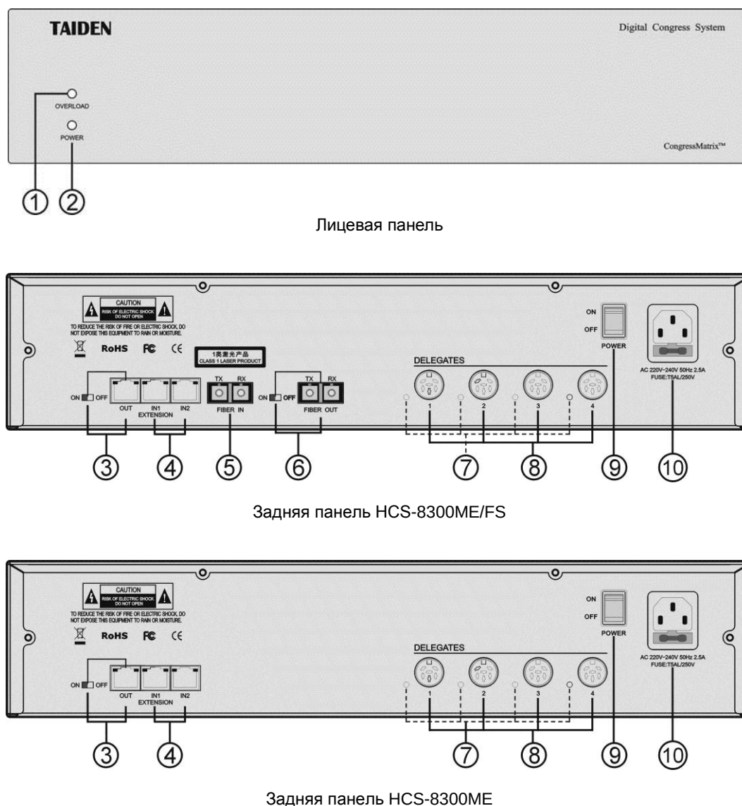
Рис. 2.2.1 Центральный блок расширения серии HCS-8300
