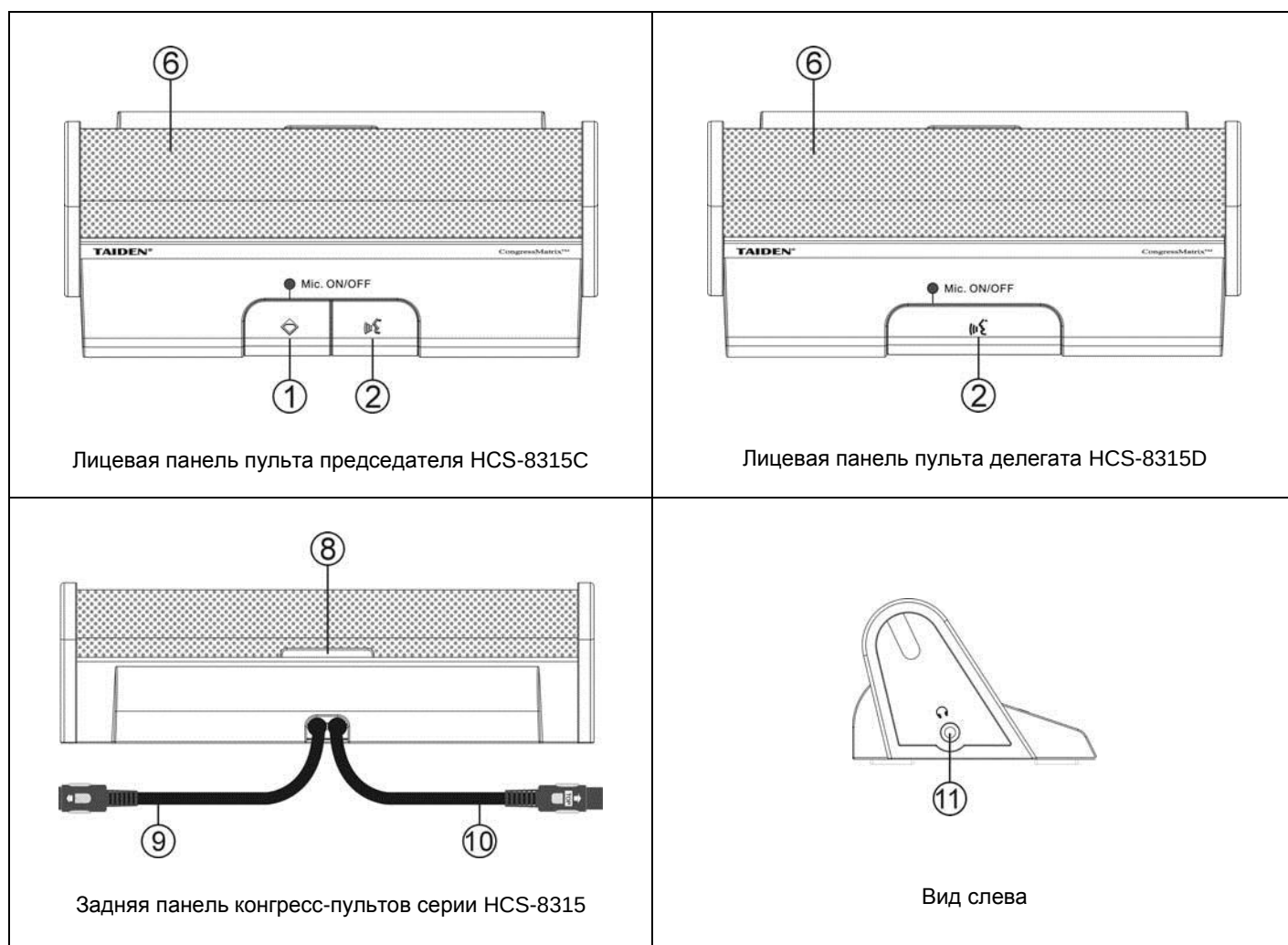
Рис. 3.2.1 Конгресс-пульта серии HCS-8315
