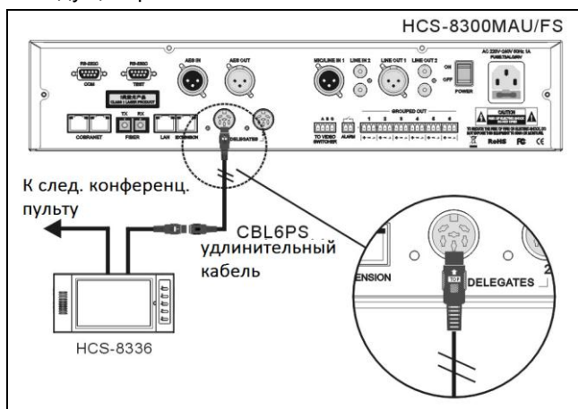
Рис. 3.4.3 Подключение монитора HCS-8336 к ЦБ/блоку расширения
