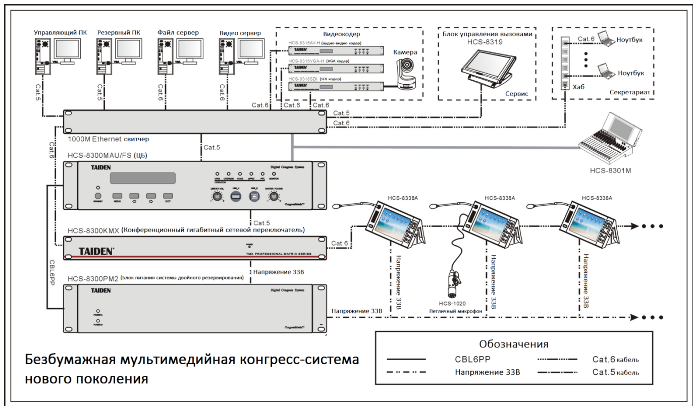
Рис. 1.1.4а Схема подключения безбумажной мультимедийной конгресс-системы нового поколения серии HCS-8338
