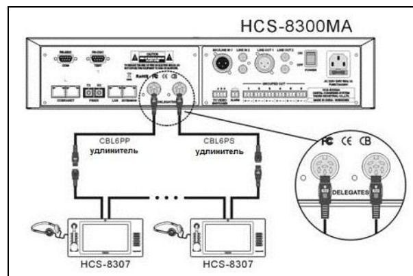
Рис. 2.1.6 Топология замкнутого гирляндного соединения
