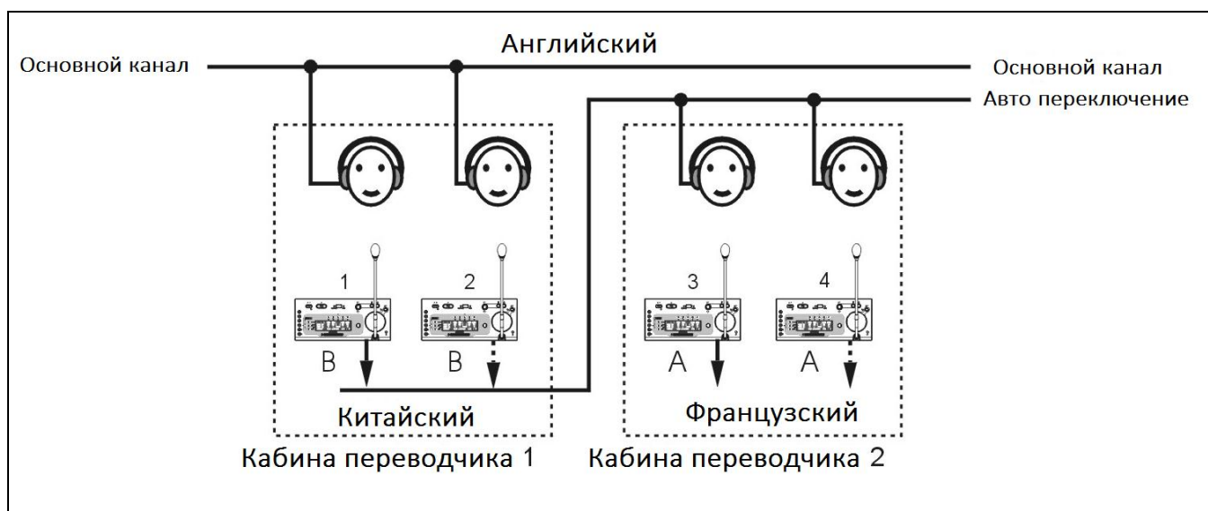
Рис. 4.4.2 Двухступенчатый перевод
