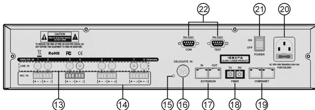
Задняя панель HCS-8300MIA/FS
