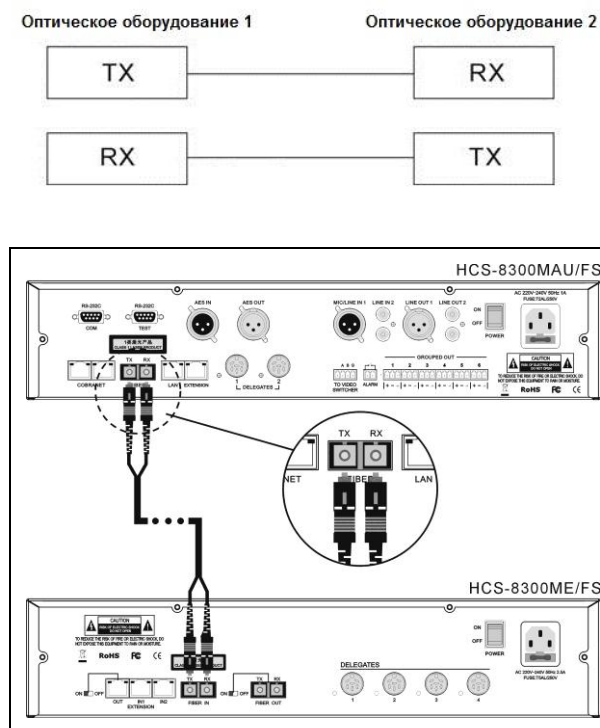
Рис. 2.8 Соединение двух центральных блоков через оптоволоконный интерфейс
