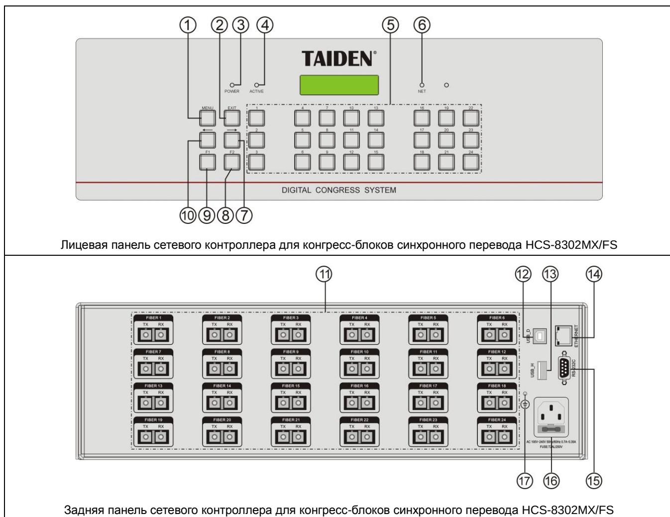
Рисунок 6.5.1 HCS-8302MX/FS Сетевой контроллер для конгресс-блоков синхронного перевода
