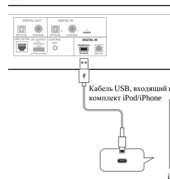
Задняя панель
