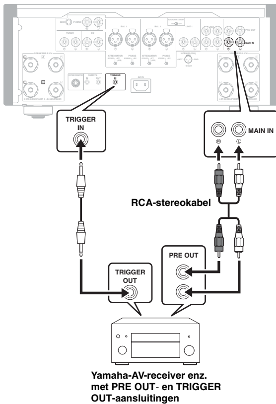
Achterpaneel van A-S3000
