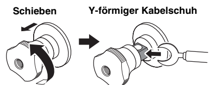
Anschlussschraube für Y-förmigen Kabelschuh: 5,0 mm Durchmesser
