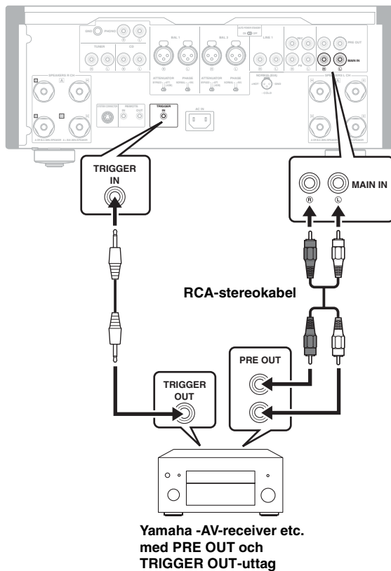
Bakpanelen på A-S3000
