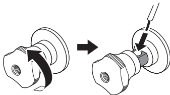
Aussparung für das Lautsprecherkabel: 6,0 mm Durchmesser
