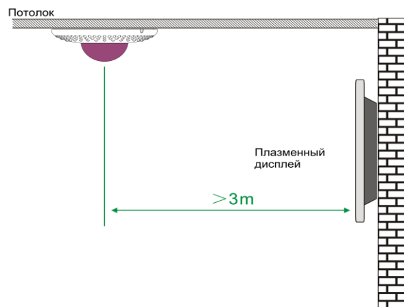
Рис. 3.9 Расположение цифрового инфракрасного ресивера (рядом с плазменным дисплеем)
