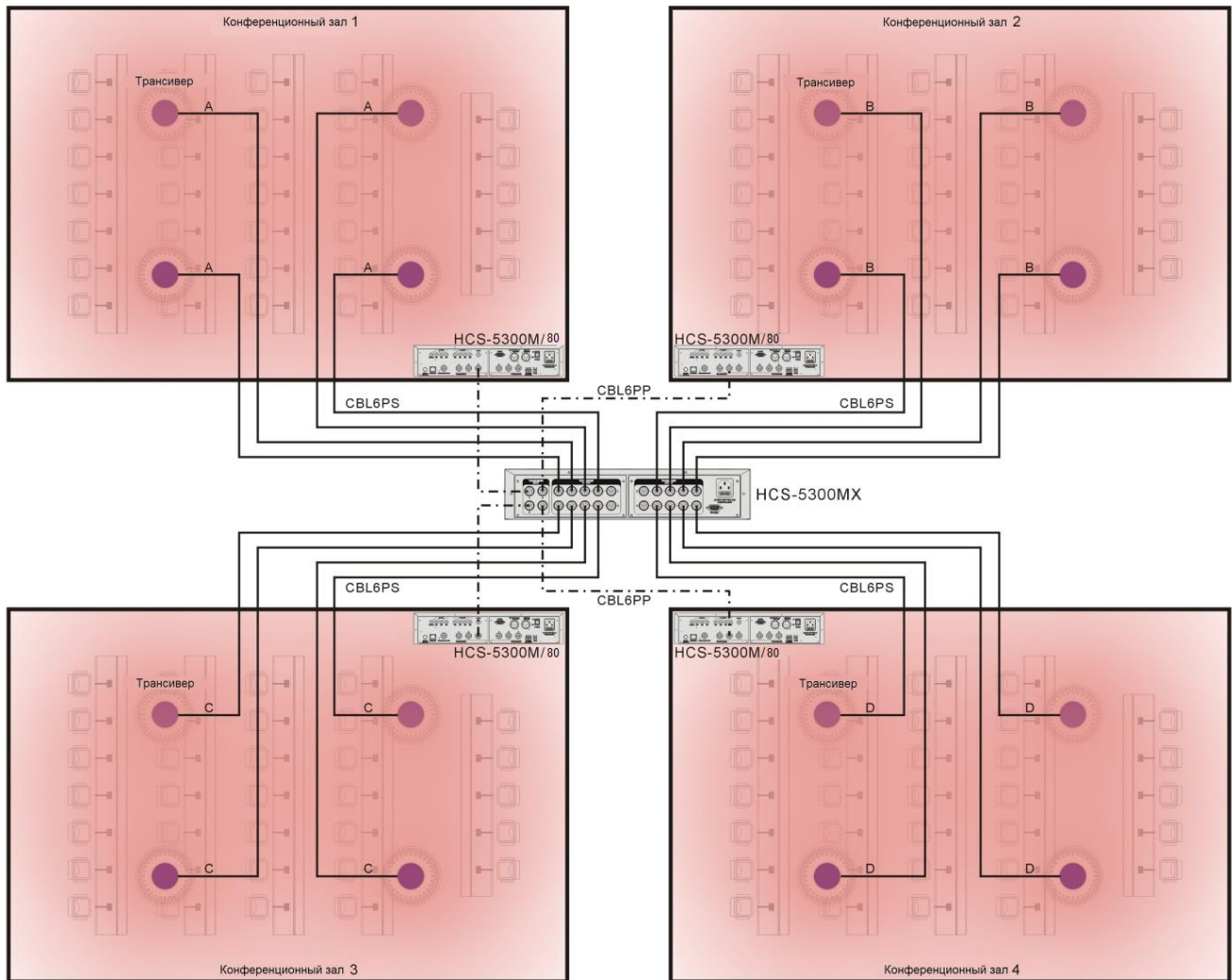
Рис.6.2 Разделение / объединение нескольких конференц-залов, вариант 1
