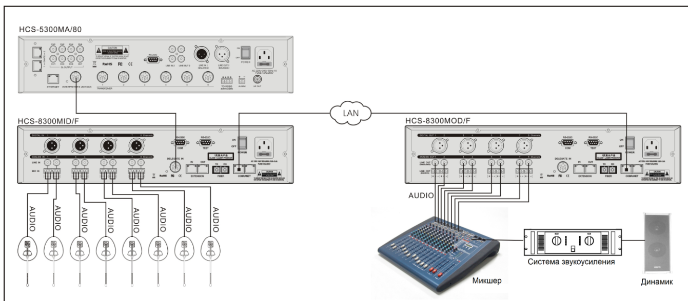
Рис. 2.8 Вариант передачи многоканального цифрового аудио сигнала с помощью устройств HCS-5300M+HCS-8300MI+HCS-8300MO
