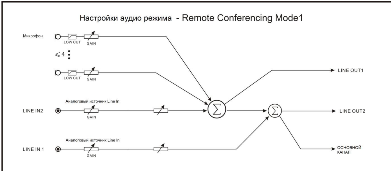
Рис. 2.14. Настройка режима аудио — Remote Conferencing Mode1 (Режим удаленной конференции 1)
