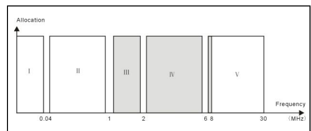
Рис. 1.3 Стандартная полоса частот системы HCS-5300/80
