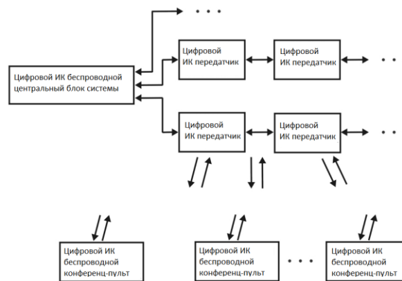
Рис. 3 Блок-диаграмма цифровой ИК конференц-системы
