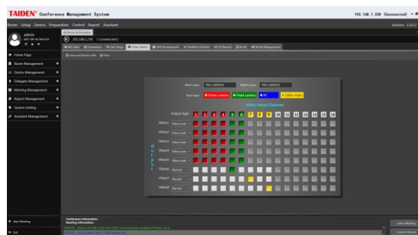
Видео матрица
