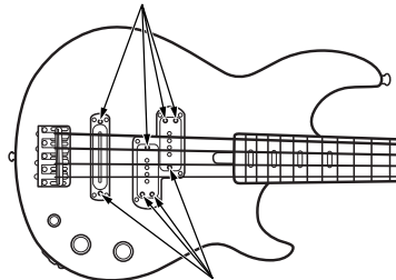
Регулировочные винты звукоснимателя
