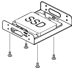
Bolt B
