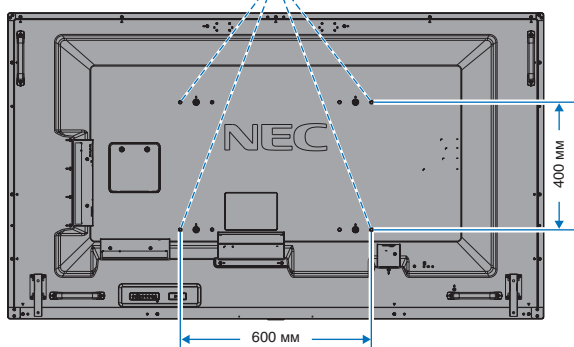
Монтажный интерфейс (M8)
