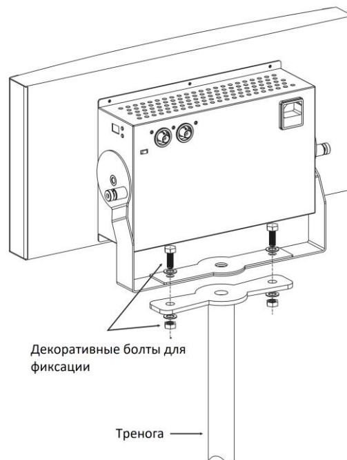
Рис. 3.9 Установка на штатив
