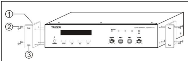
Рис. 2.2 Установка передатчика
