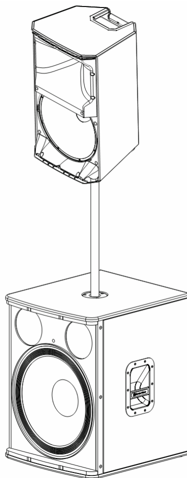
Рис. 2b...ZLX на соединительной стойке ASP-1 с сабом
