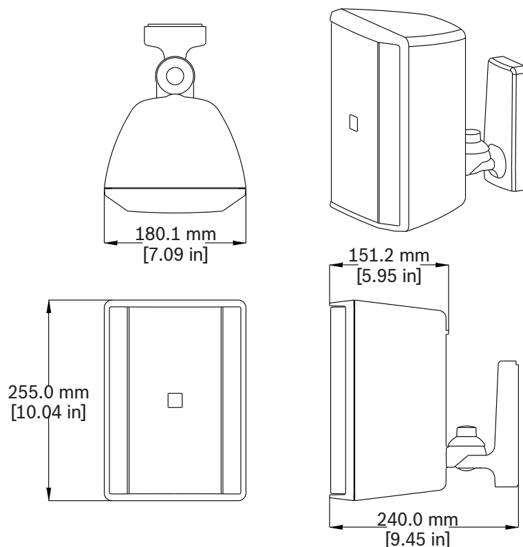
Рис. 6.3: Габариты EVID-S5.2/EVID-S5.2T
