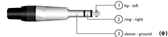
PHONES Stereo Jack
