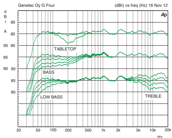
Kuva 5. "Bass"-, "treble"-, "tabletop"- ja "low bass"-säätöjen vaikutus G Four:n vapakenttävästeeseen.
