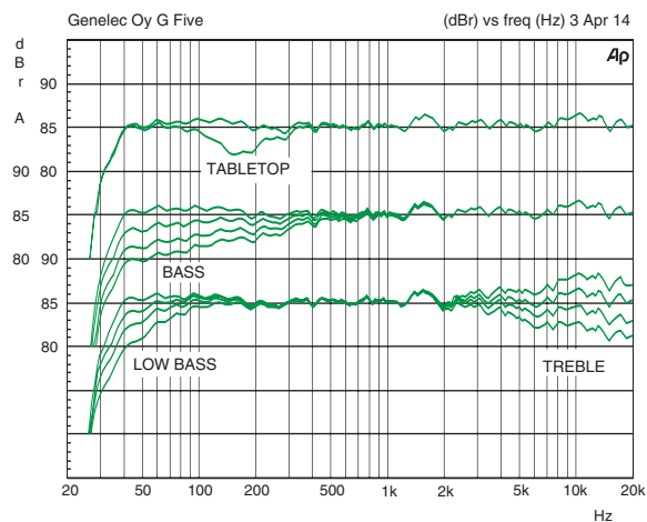
Kuva 7. "Bass"-, "treble"-, "tabletop"- ja "low bass"-säätöjen vaikutus G Five:n vapakenttävästeeseen.
