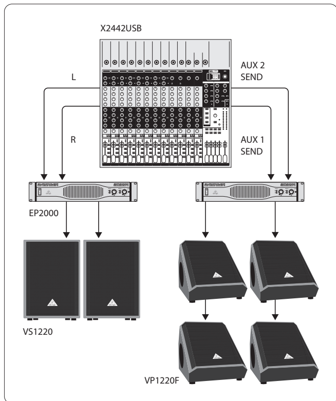
Фиг. 5.2: Стерефонический режим с полным частотным диапазоном и напольными мониторами
