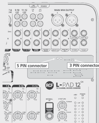
5-Pin-Verbinder
